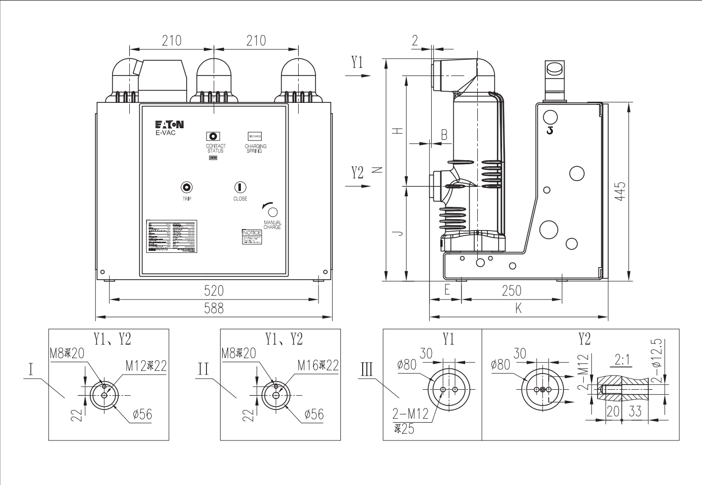
E-VAC 固定式真空断路器外形图 (210相间距)
